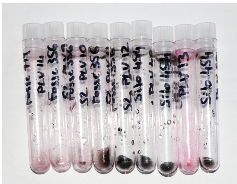
Figure 3. Les extractions permettent l'obtention de concentrés polliniques (cf. photographie).
