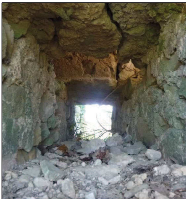
Photo 20 : Emplacement des poutres dans la maçonnerie intérieure de la tour (UC 1, UC 2)
