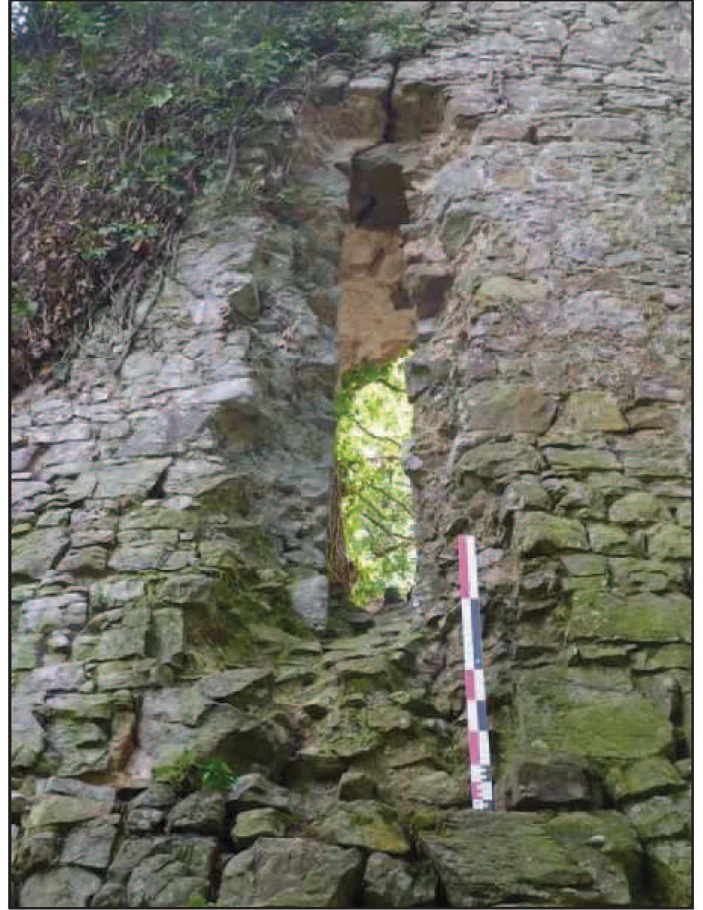
Photo 25 : Archère UC 3 dans parement extérieur
